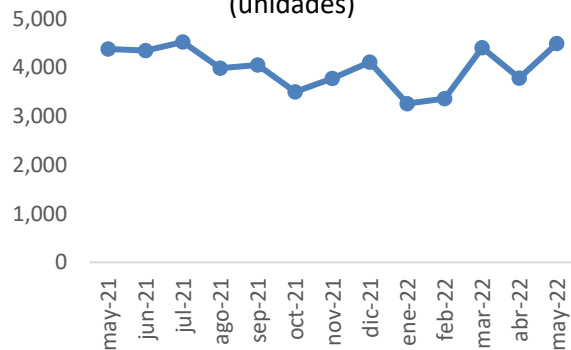
Venta de vehículos híbridos y eléctricos (unidades)
